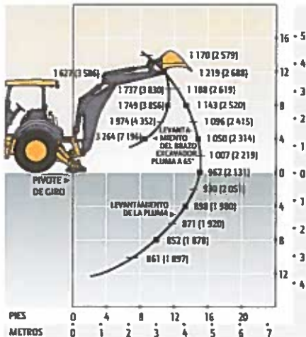
LEVANTAMIENTO ESTÁNDAR Con brazo excavador estándar
